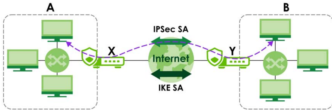
Figure 78 VPN: IKE SA and IPsec SA
